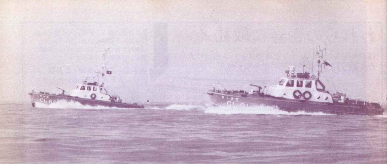
雁行する海上保安庁の15メートル型巡視艇「こまかせ」「きくかせ」。ともに満載排水量19トンで、1971年建造。(池田 良穂)
