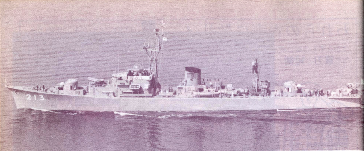
護衛艦「きたかみ」。「いすず」型の3番艦で、昭和39年就役。同型艦「おおい」と第32護衛隊を編成している。(津村 豊)
