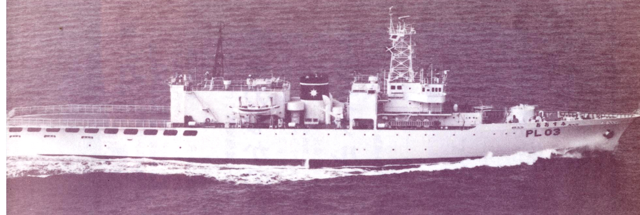
同じくヘリコプター搭載巡視船の第3船“おおすみ”。常備排水量3,643トン。三井造船玉野事業所で昭和54年10月18日竣工。
