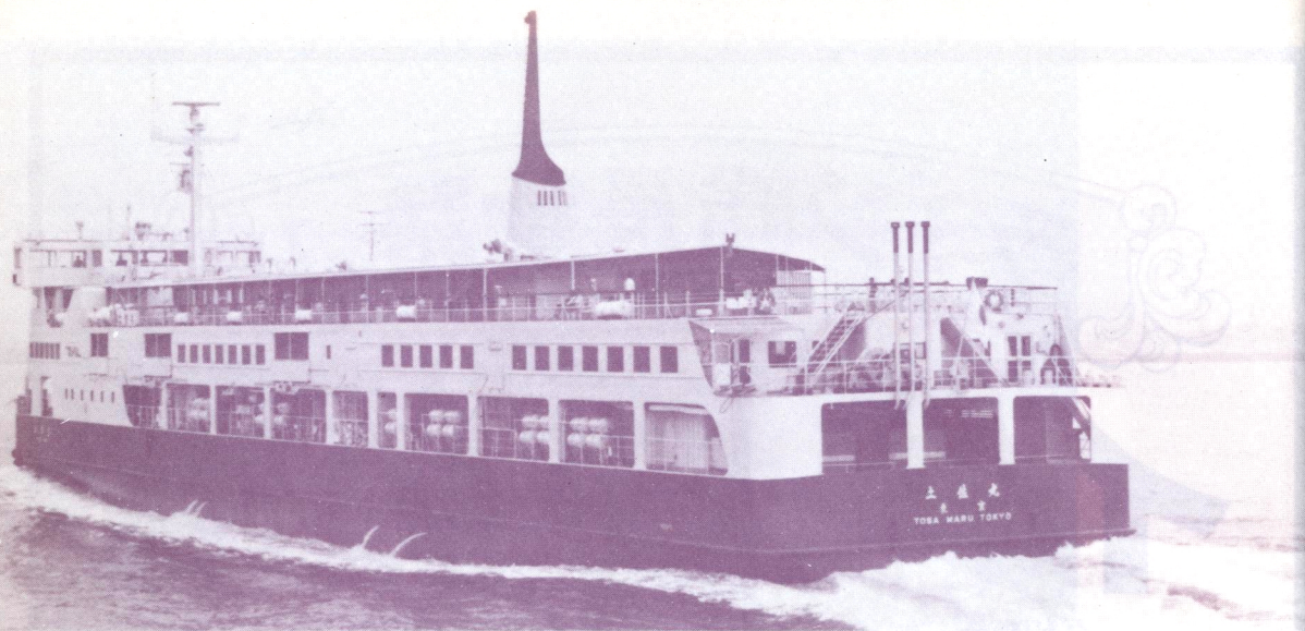
国鉄宇高鉄道連絡船土佐丸。3,083総トン、速力16.3ノット、船客定員1,800名、15トン貨車2両積載。1966年竣工。(迫口 充久)
