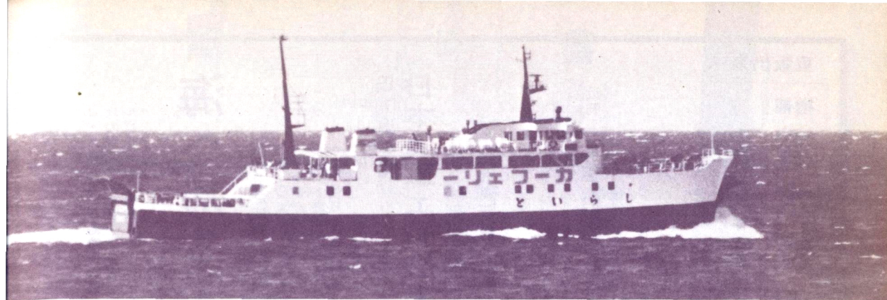
駿河湾カーフェリーの田子の浦～土肥航路に就航するフェリー「しらいと」。490総トン、航海速度14ノット、1970年建造。
