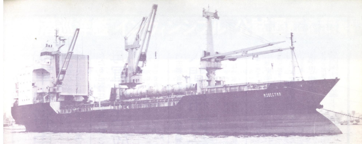
右舷前方から見たイズベスチャ。12,600重量トン、全長133.3メートル、幅20.5メートル、速力16ノット。(橋本 広)
