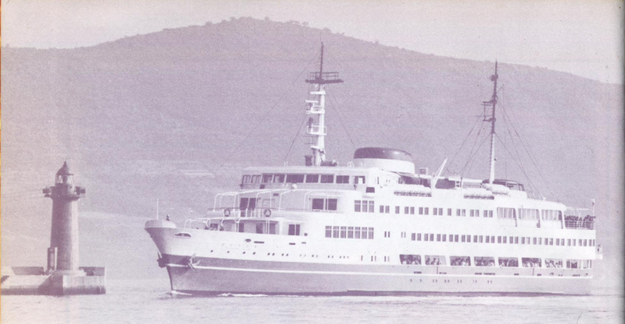
関西汽船の阪神～別府航路客船むらさき丸。総トン数2,991トン、速力18.5ノット、1960年竣工。(迫口 充久)
