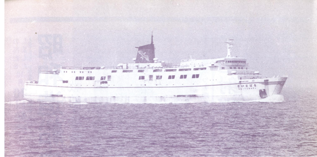
日本カー・フェリーの神戸～日向航路フェリー“さいとばる”6,496総トン、速力21.5ノット、1972年建造。(佐藤 善平)
