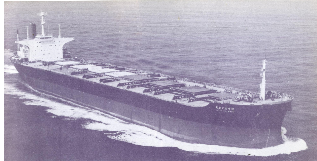
大阪商船三井船舶と大阪船舶共有の鉱石運搬船おせあにあ丸。住友重機械工業追浜造船所で11月30日竣工。
