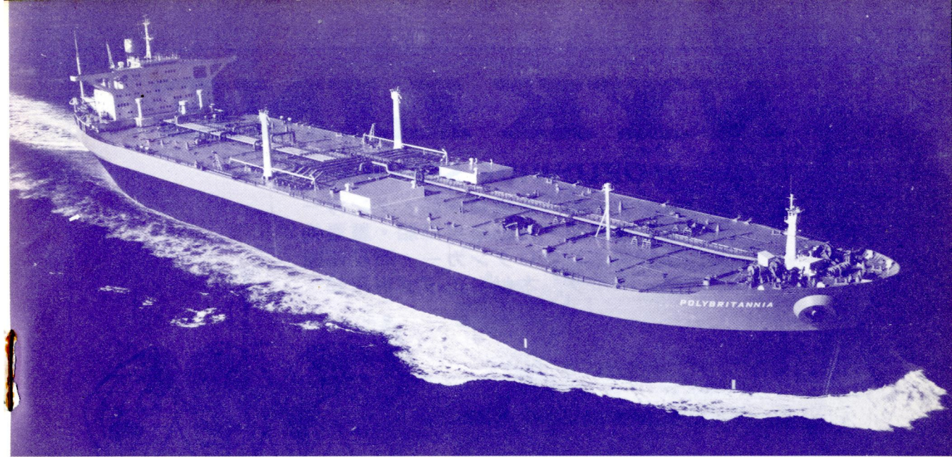
ノルウェー向け輸出油槽船ポリブリタニアPolybritannia。三井造船千葉造船所で11月26日竣工。268,960重量トン。
