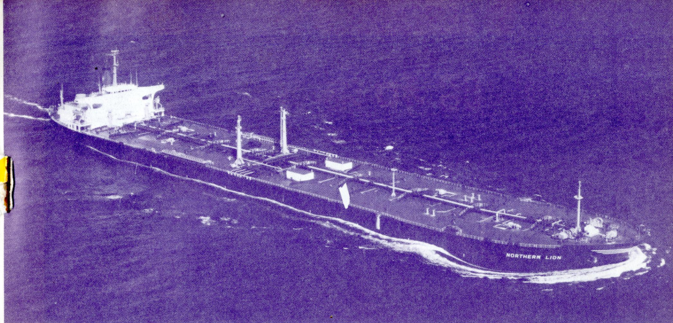
リベリア向け輸出油槽船ノーザン・ライオンNorthern Lion。日立造船堺工場で10月25日竣工。264,829重量トン。
