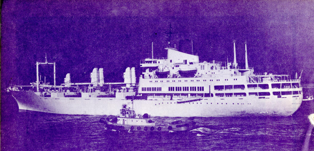
神戸港における巡視見本市船“新さくら丸”。13,900総トン，航海速力20.6ノット，1972年竣工。市栄 正樹
