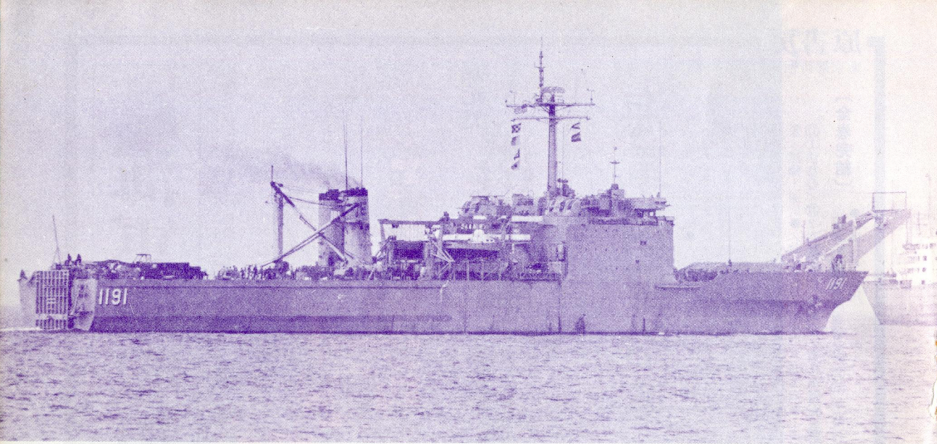
米海軍の戦車揚陸艦ラシーンRacine LST-1191。新鋭ニューポート級の一艦で、去る7月27日、神戸を出港中の姿。
