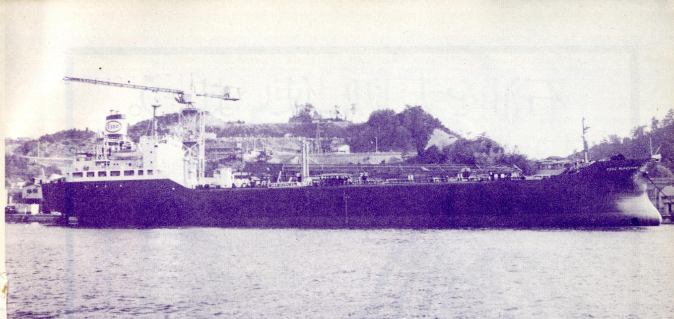
リベリア向け油槽船エッソ・ムカイシマEsso Mukaiishima。日立造船向島工場で3月18日竣工。22,374重量トン。
