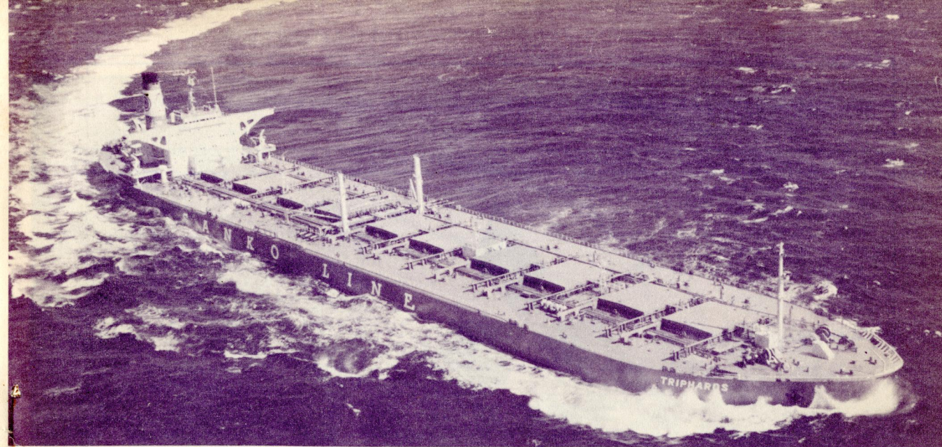
リベリア向け輸出鉱油槽船トリファロスTripharos。日立造船因島工場で4月4日竣工。162,385重量トン。
