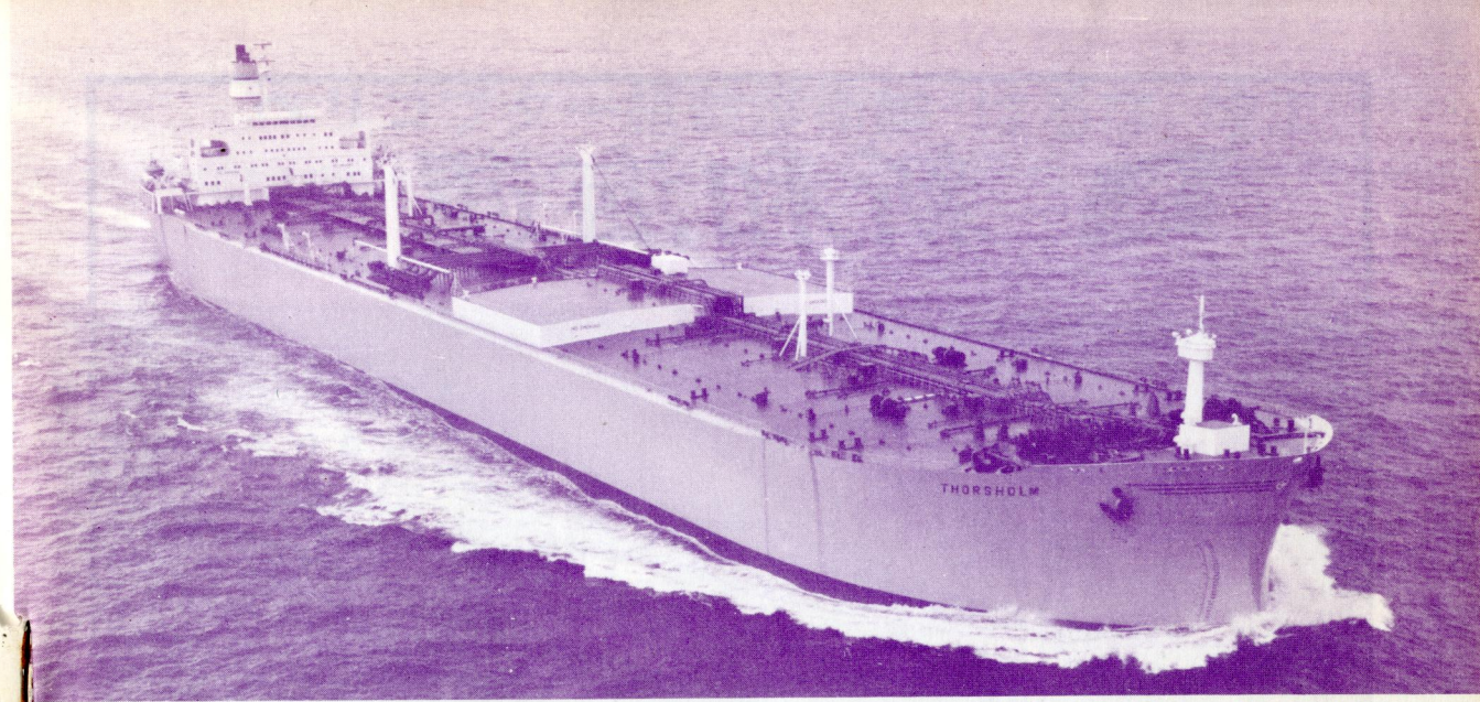
ノルウェー向け大型油槽船トールスホルムThorsholm。三井造船千葉造船所で2月15日竣工。279,810重量トン。
