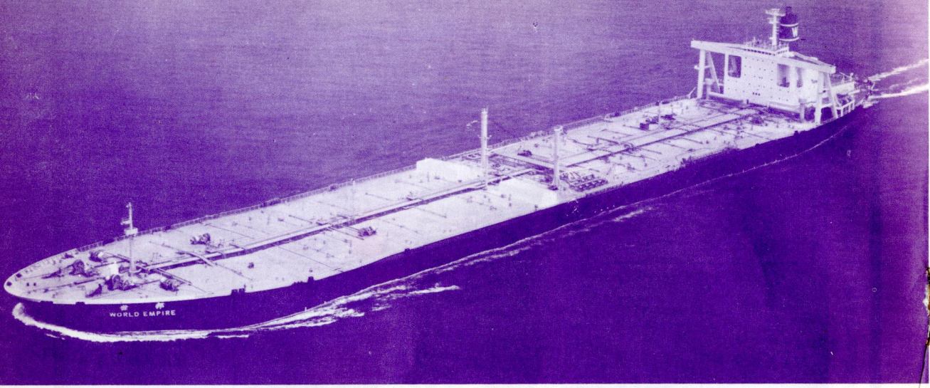
パナマ向け輸出タンカー“ワールド・エンパイア” World Empire。川崎重工坂出工場で7月18日竣工。228,172重量トン。
