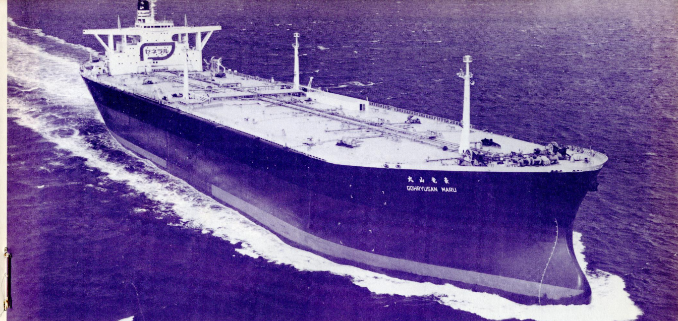
大阪商船三井船舶・ゼネラル海運共有の油槽船豪竜丸。三井造船千葉造船所で8月7日竣工。世界最大のディーゼル装備。
