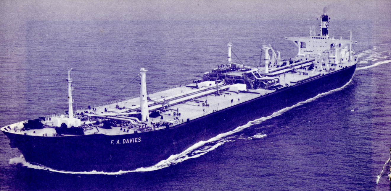
リベリア向け輸出油槽船兼貯油船F.A.デイビス。三菱長崎造船所で5月12日竣工。229,516重量トン、航海速力15.9ノット。
