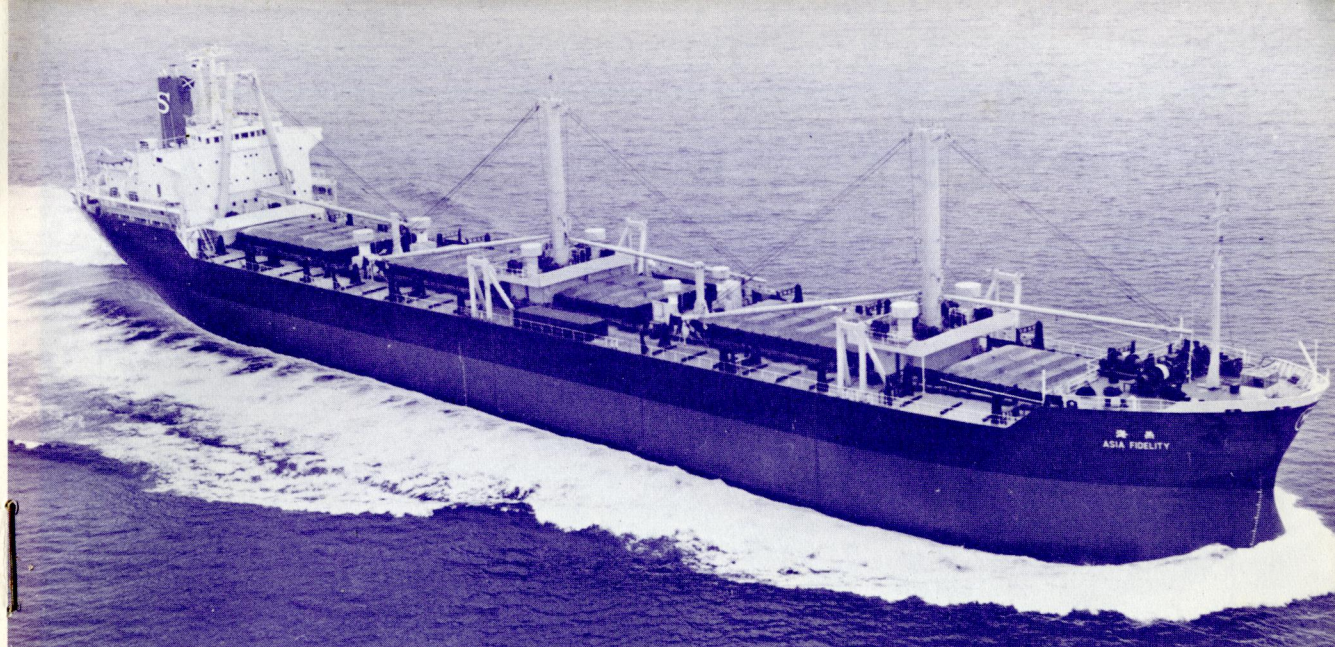
香港向け自動車兼撤積貨物船エイシャ・フィデリティ。佐世保重工で6月14日竣工。25,111重量トン、航海速力15.0ノット。
