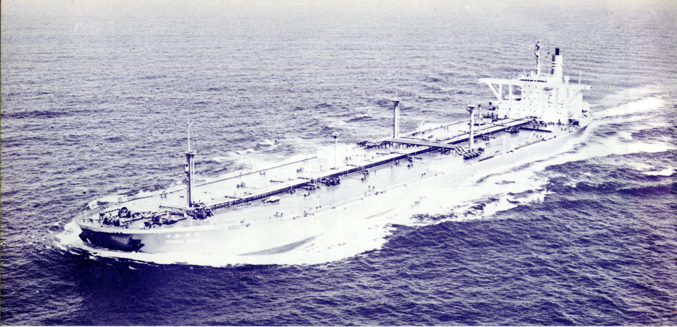
日本郵船・太平洋海運のタンカー“十和田丸”。三菱重工長崎造船所で9月22日竣工。227,290重量トン、航海速力16ノット。
