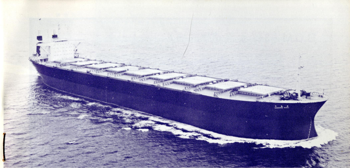
第一中央汽船の大型撒積貨物船“鹿島丸”。住友重機械工業浦賀造船所で9月30日竣工。120,174重量トン、最大速力17.5ノット。
