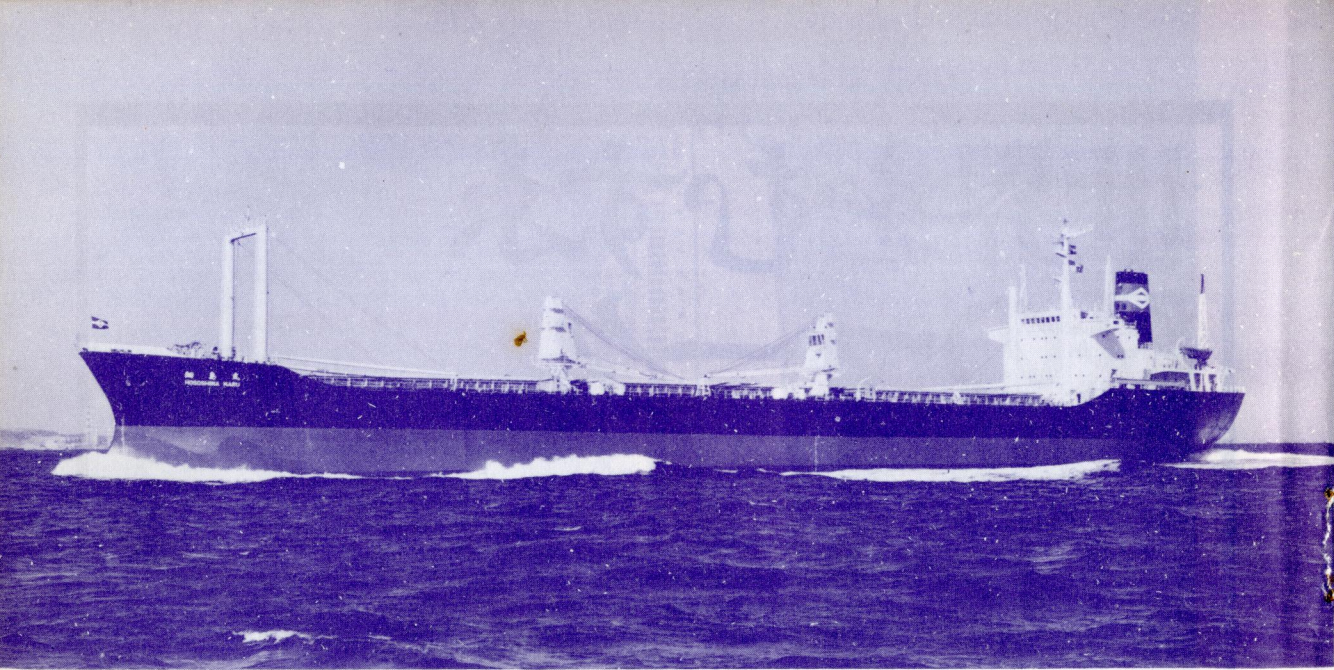
第一中央汽船のニッケル鉱石専用船細島丸。住友重機械工業浦賀造船所で2月21日竣工。23,660重量トン、航海速力14.9ノット。
