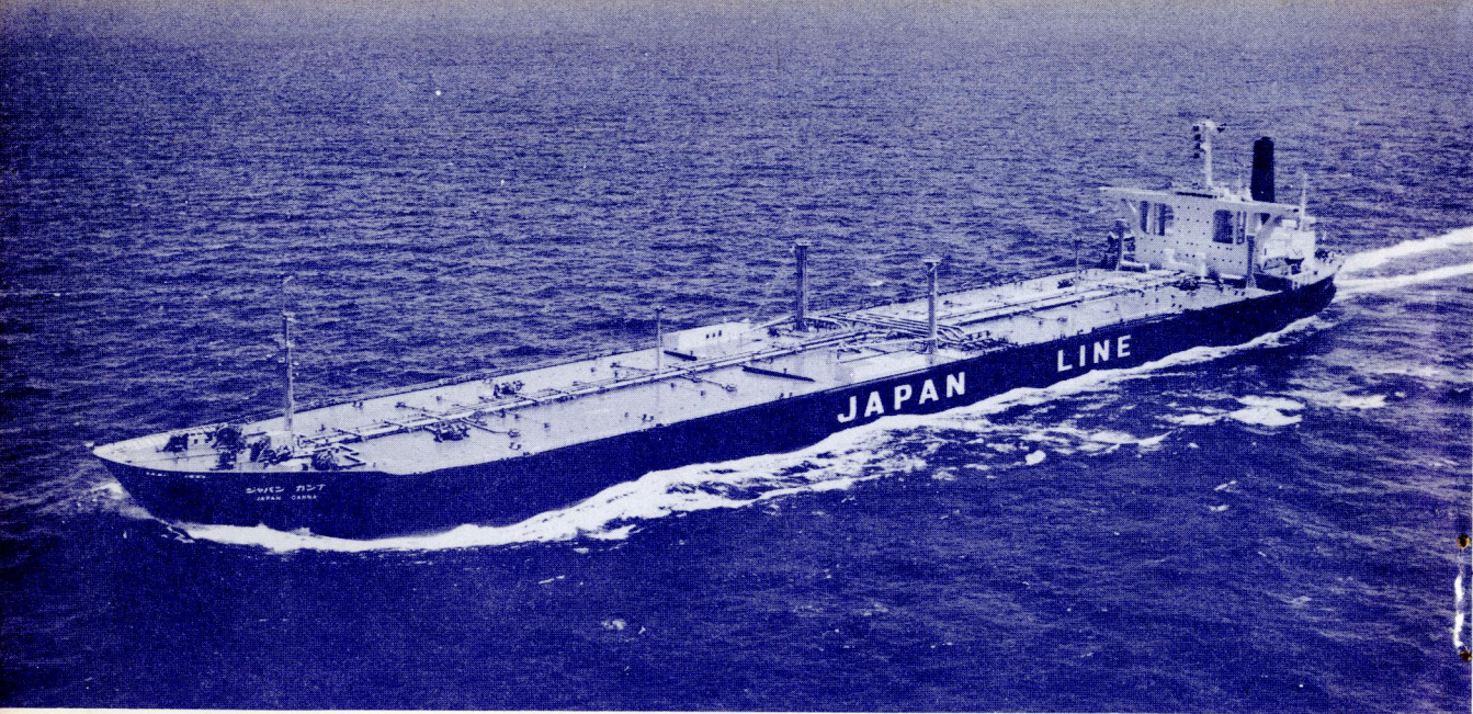
ジャパン・ラインの油槽船ジャパン・カンナ。三菱重工業長崎造船所で6月25日竣工。210,243重量トン、航海速力16.2ノット。
