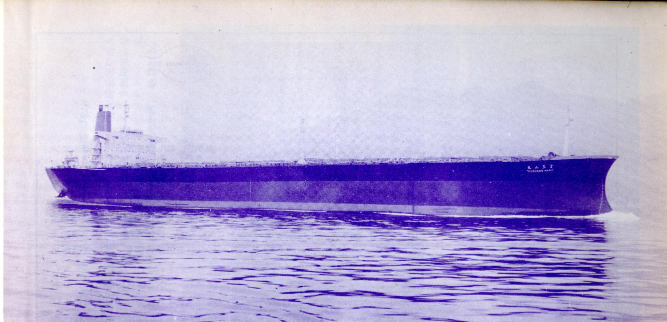
大阪商船三井船舶の鉱石兼油運搬船富王山丸。日立造船因島工場で6月28日竣工。113,369重量トン、満載航海速力14.9ノット。
