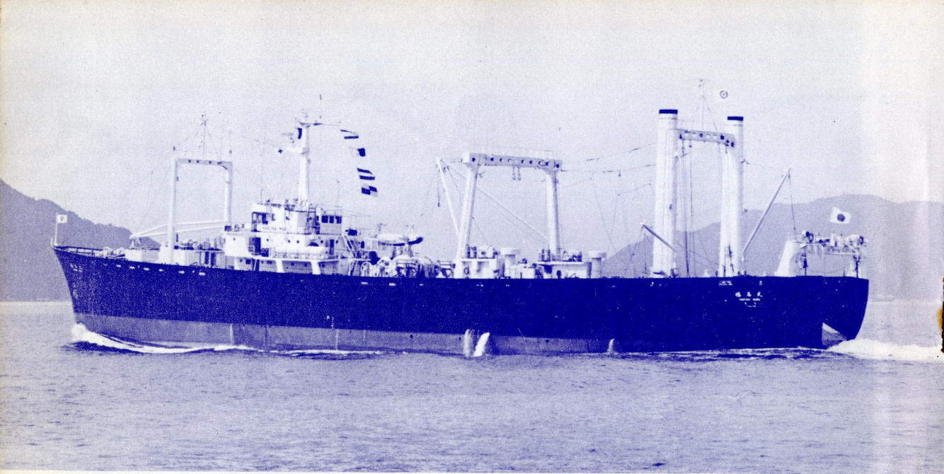
日本水産の大型船尾トロール漁船標名丸。日立造船向島工場で昨年11月5日竣工。4,039.9総トン、満載航海速力13.75ノット。
