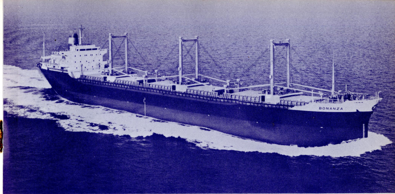
リベリア向け撒積貨物船“ボナンザ” Bonanza。三井造船藤永田造船所で10月2日竣工。24,930重量トン、公試速力16.5ノット。
