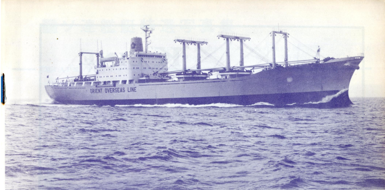
中華民国向けセミ・コンテナ船“亦雲”。浦賀重工浦賀造船工場で10月5日竣工。去る4月完成した凌雲の姉妹船である。
