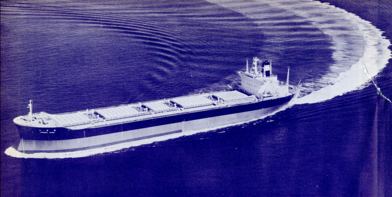
第一中央汽船の撒積貨物船“小倉丸”。三井造船玉野造船所で9月19日竣工。45,834重量トン、満載航海速力14.95ノット。
