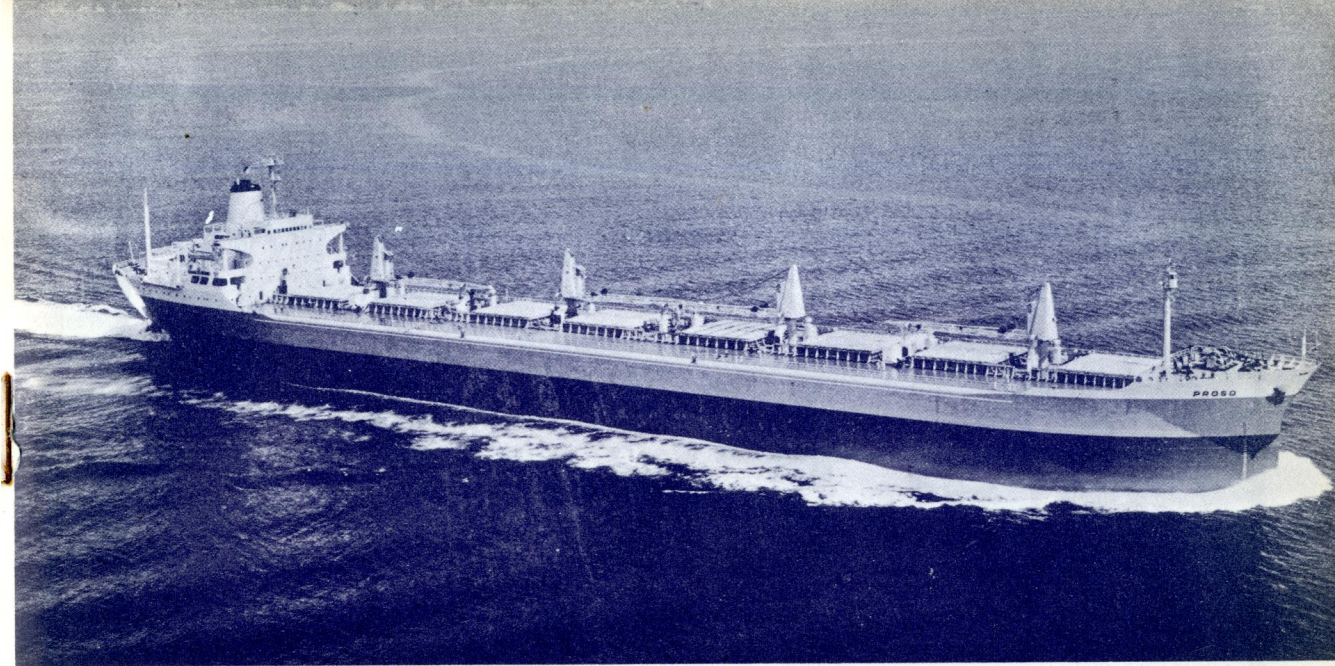
ギリシア向け輸出搬積貨物船プロソProso。三菱重工広島造船所で7月25日竣工。66,300重量トン、最高速力16.9ノット。
