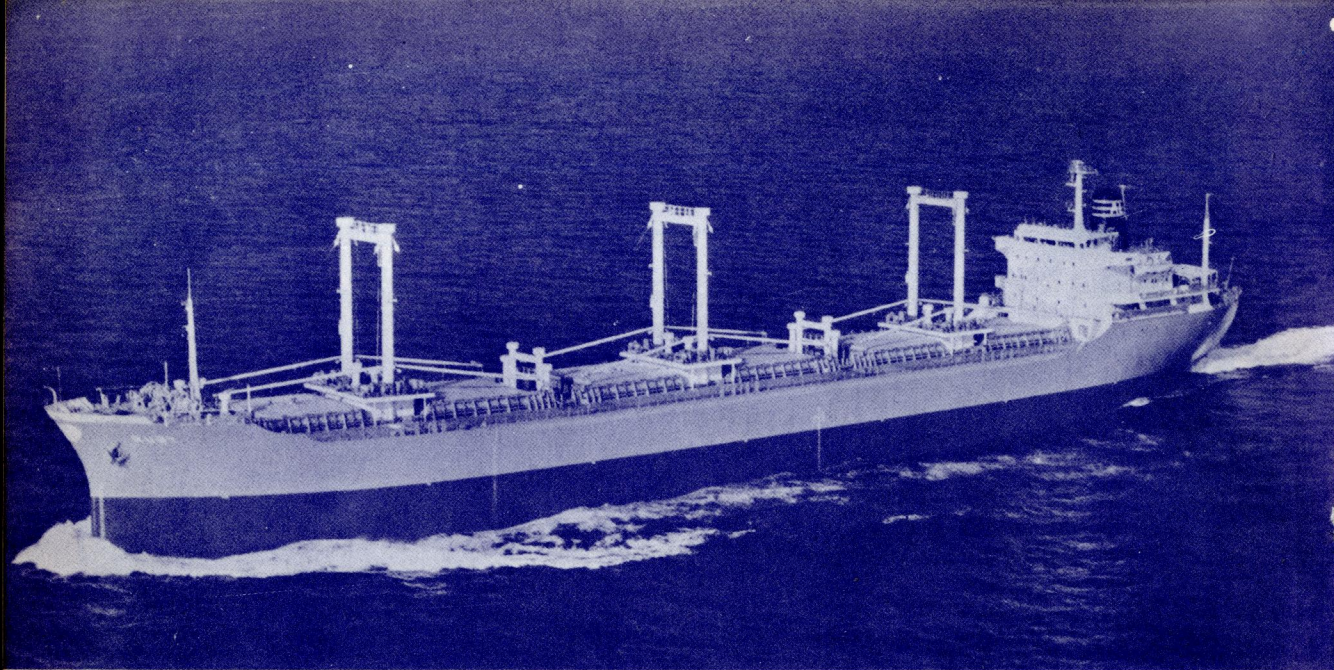
リベリア向け輸出撒積貨物船ルビ Ruby。三井造船藤永田造船所で7月15日竣工。26,883重量トン、航海速力15.25ノット。
