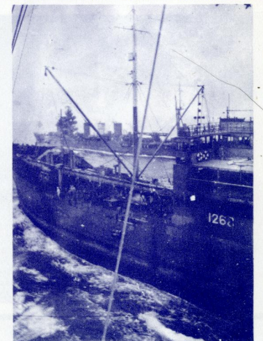
「アリエーション」作戦で、洋上補給中の給油艦「日本丸」。満腹して離れて行くのは軽巡洋艦「阿武隈」
