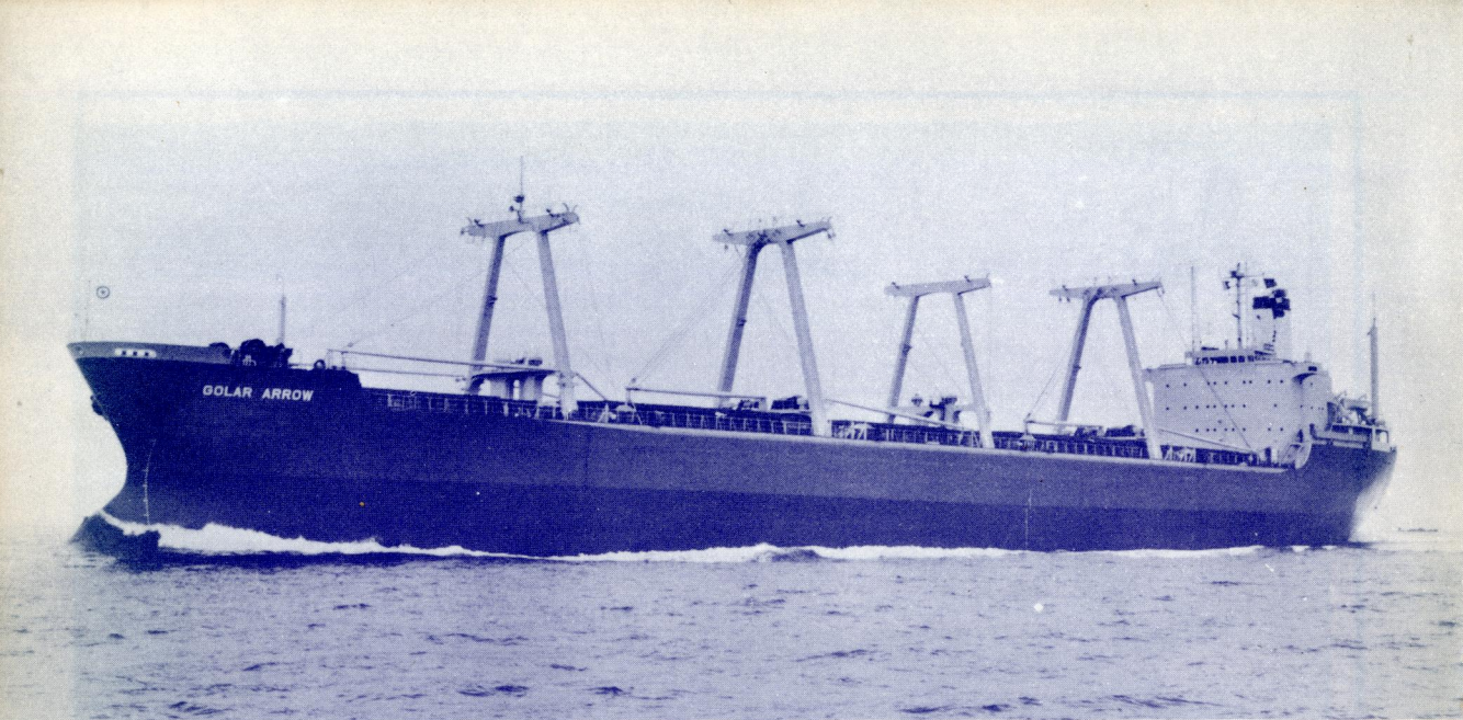
リベリア向け撒積貨物船ゴラー・アローGolar Arrow。三菱重工神戸造船所で10月27日竣工、26,139重量トン。
