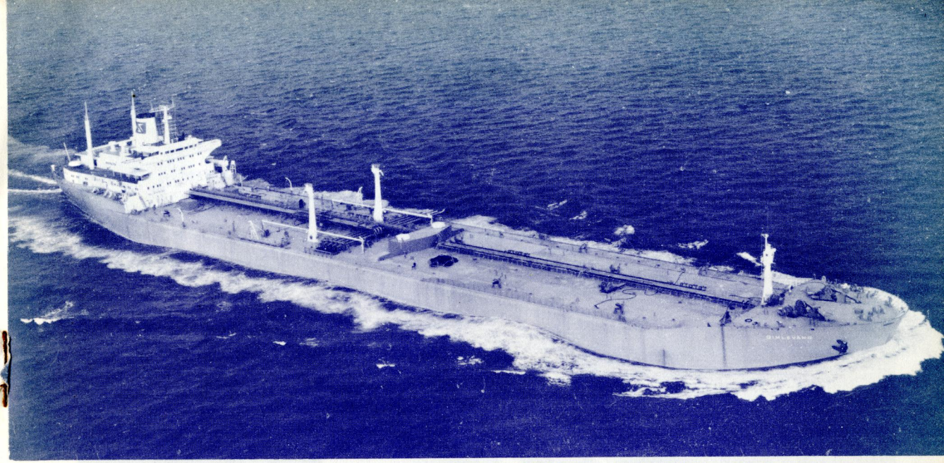
ノルウェー向け油槽船ギムレバンク Gimlevang。三井玉野造船所で10月12日竣工，79,582重量トン，満載航海速力15.9ノット。
