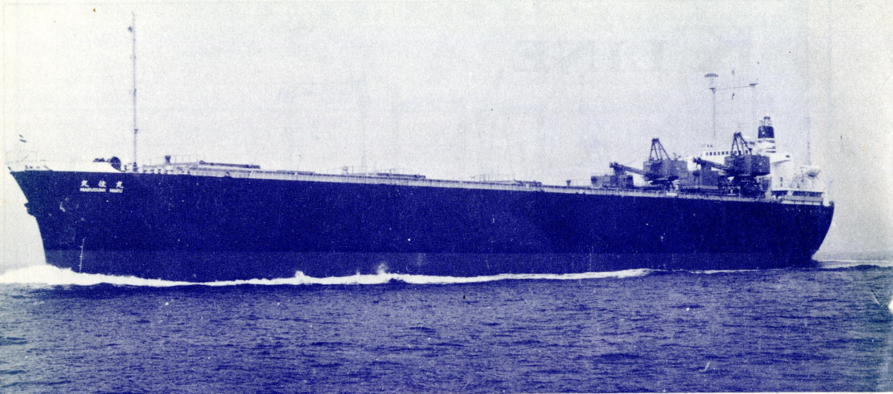
日本郵船・八馬汽船共有の木材チップ専用船丸住丸。浦賀重工で10月6日竣工，24,208重量トン，満載航海速力13.9ノット。
