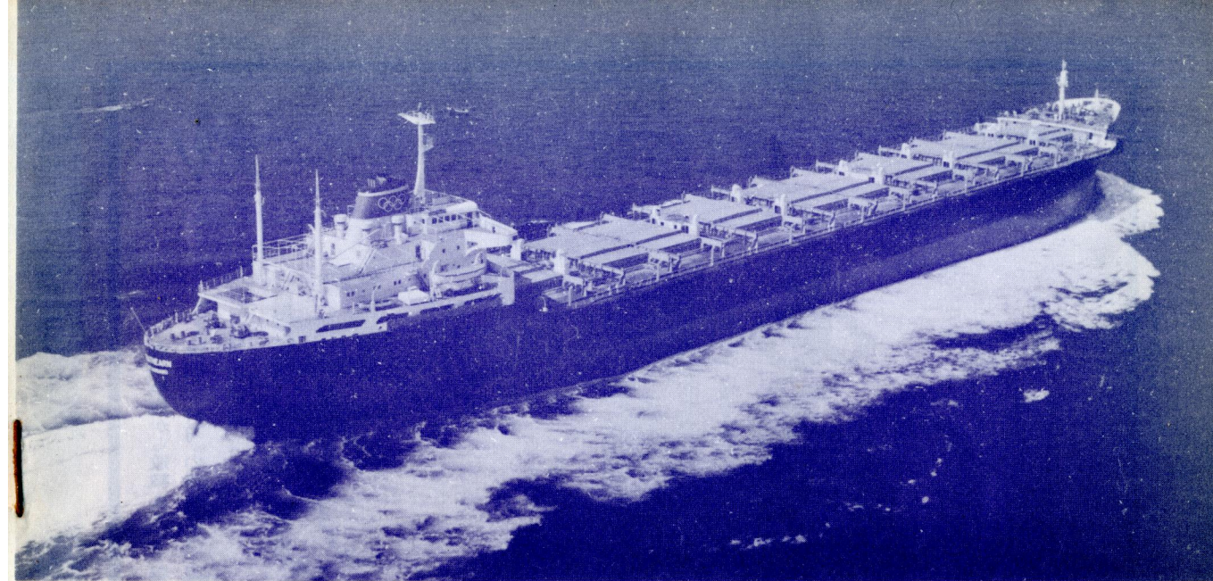
ノルウェー向け撒積貨物船ストラサーン (Strathearn)。浦賀重工浦賀造船工場で3月25日竣工、52,288重量トン。
