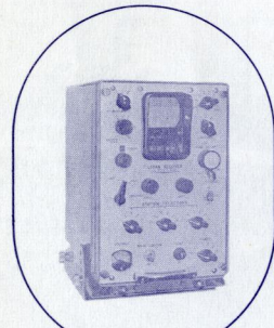
LR-700型 ロランC-A受信機
