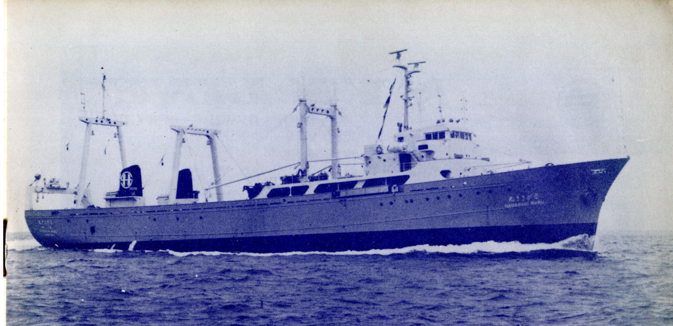
長崎県南方漁業会社のトロール漁船“ながさき丸”。7月15日林業造船下関造船所で竣工，2,202総トン，航海速力13.25ノット。
