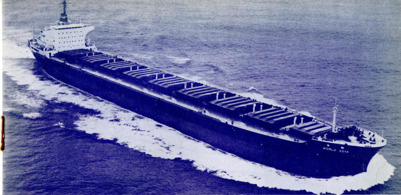
香港向け輸出搬積貨物船ワールド・ソヤ World Soya。佐世保重工佐世保造船所で7月21日竣工、69,422重量トン。
