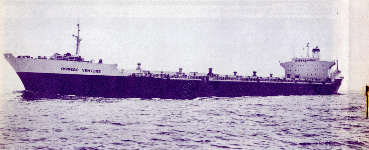
リベリア向け鉱石運搬船オスエゴ・ベンチュア Oswego Venture。三菱重工神戸造船所で5月27日竣工、52,554重量トン。
