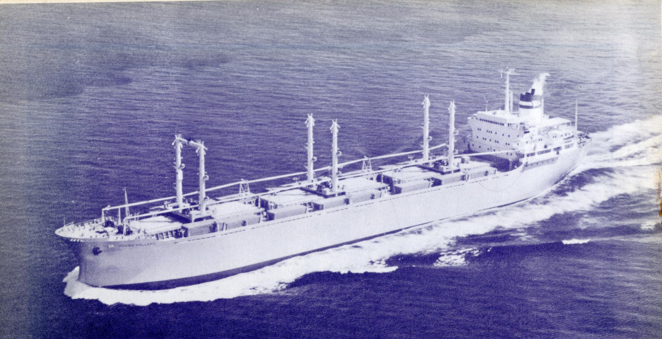
ノルウェー向け輸出搬積貨物船ホッグ・マラード(Høegh Mallard)。川崎重工で4月12日竣工、22,300重量トン。
