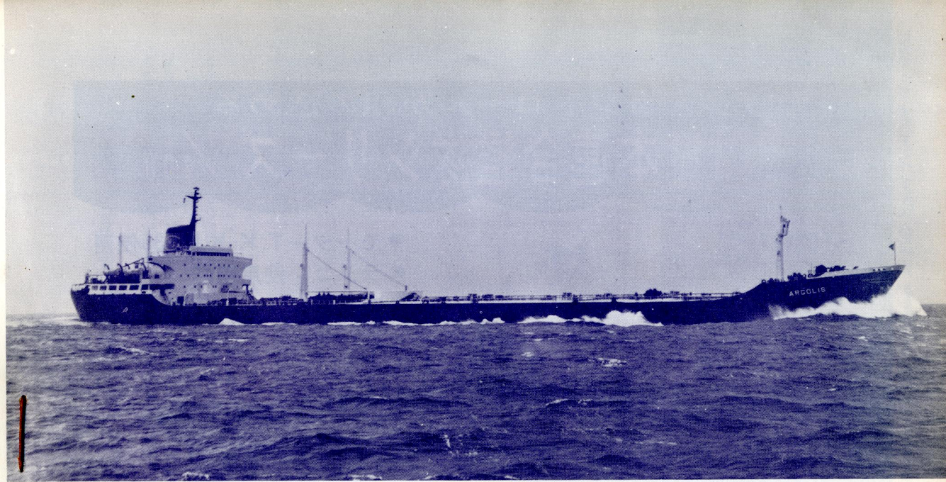
リベリア向け輸出タンカー“アルゴリス” Argolis。浦賀重工浦賀造船工場で昨年12月21日竣工，50,881重量トン。
