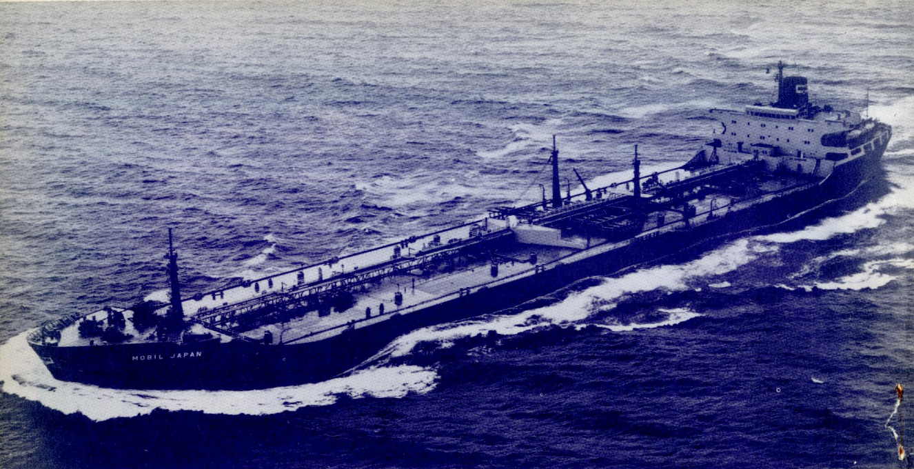
アメリカ向け輸出タンカー“モービル・ジャパン” Mobil japan。三井造船玉野造船所で7月22日竣工，82,436重量トン。
