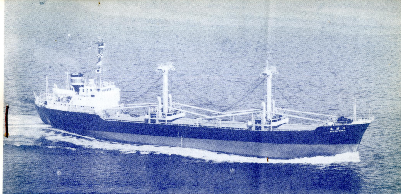
東京船舶の木材運搬船三浦丸。石川島播磨重工相生第一工場で2月23日竣工。5,187重量トン、航海速力12.1ノット。
