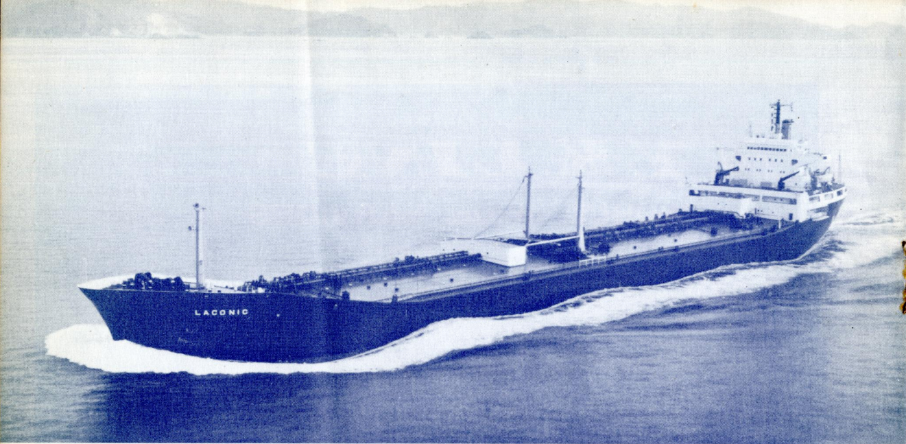
パナマ向け輸出油槽船ラコニックLaconic。石川島播磨重工相生第一工場で2月12日竣工。56,405重量トン、航海速力16ノット。
