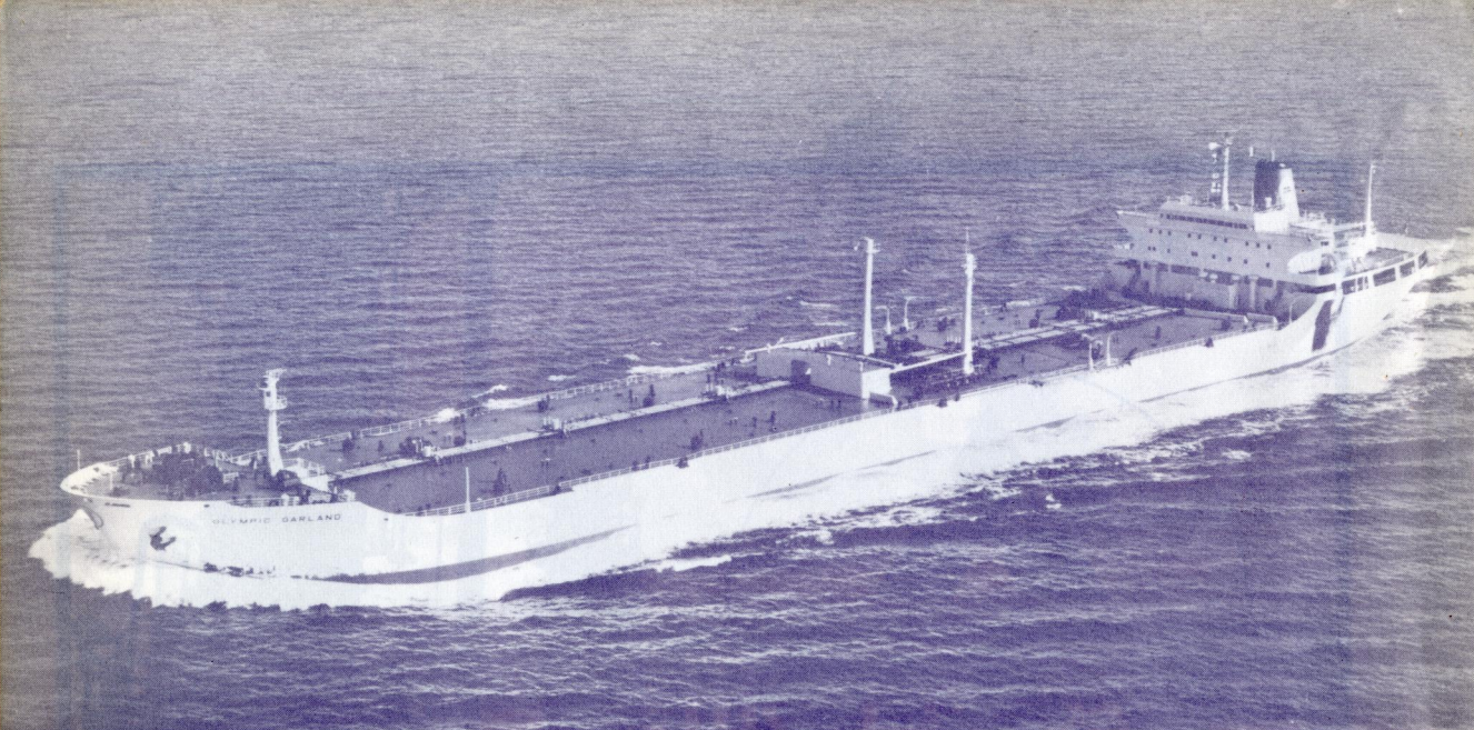
パナマ向け輸出油槽船オリンピック・ガーランド。去る3月17日石川島播磨重工相生第一工場で竣工。73,986重量トン
