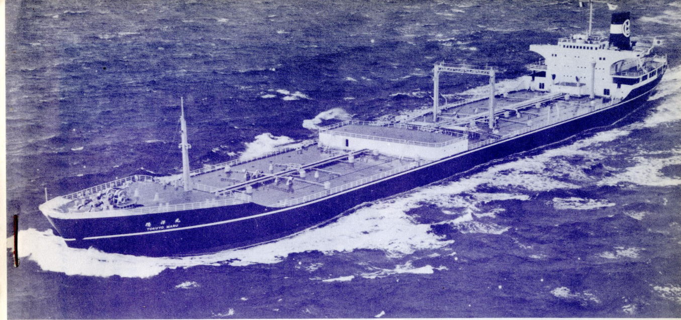
大洋商船の油槽船徳洋丸。佐世保重工佐世保造船所で昨年1月31日竣工。51,561重量トン、航海速力16ノット。
