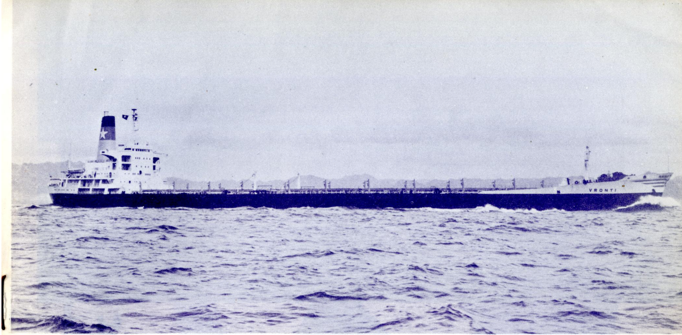
リベリア向け輸出鉱石兼油運搬船ブロンティ Vronti。三菱日本重工横浜造船所で4月14日竣工。51,800重量トン、速力15.60ノット。
