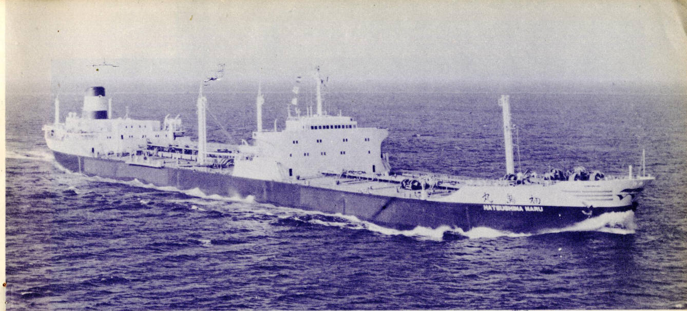
東燃タンカー向け油送船初島丸。7月13日に石川島播磨重工相生第一工場で竣工した超大型油送船で、大巾に自動化されてる。
