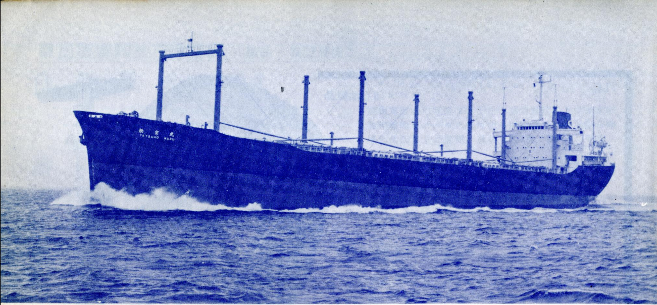
新和海運の鉱石運搬船「鉄宝丸」。浦賀重工浦賀工場で昨年11月26日竣工。28,299.5重量トン、航海速力13.8ノット。
