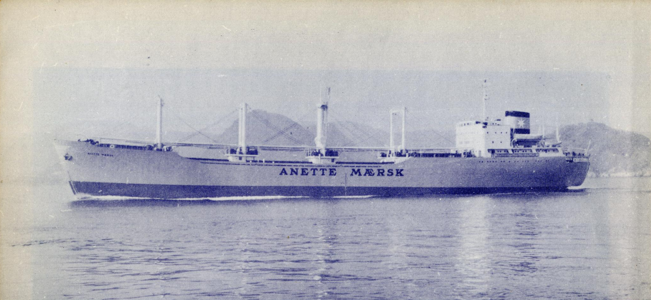
デンマーク向け貨物船「アネッテ・マースク」Anette Maersk。8月15日三井造船玉野造船所で完成。12,300重量トン、16.4ノット。
