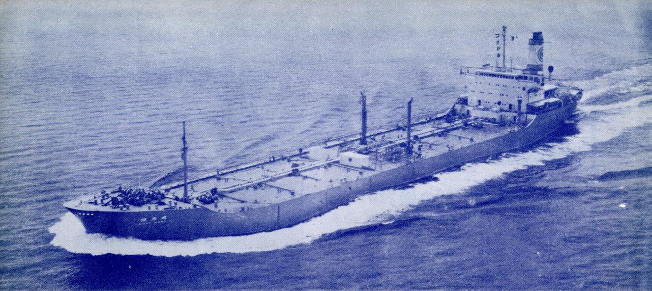
三光汽船の油槽船“銀光丸”。石川島播磨重工相生工場で9月10日完成。34,318重量トン、航海速力16.0ノット。
