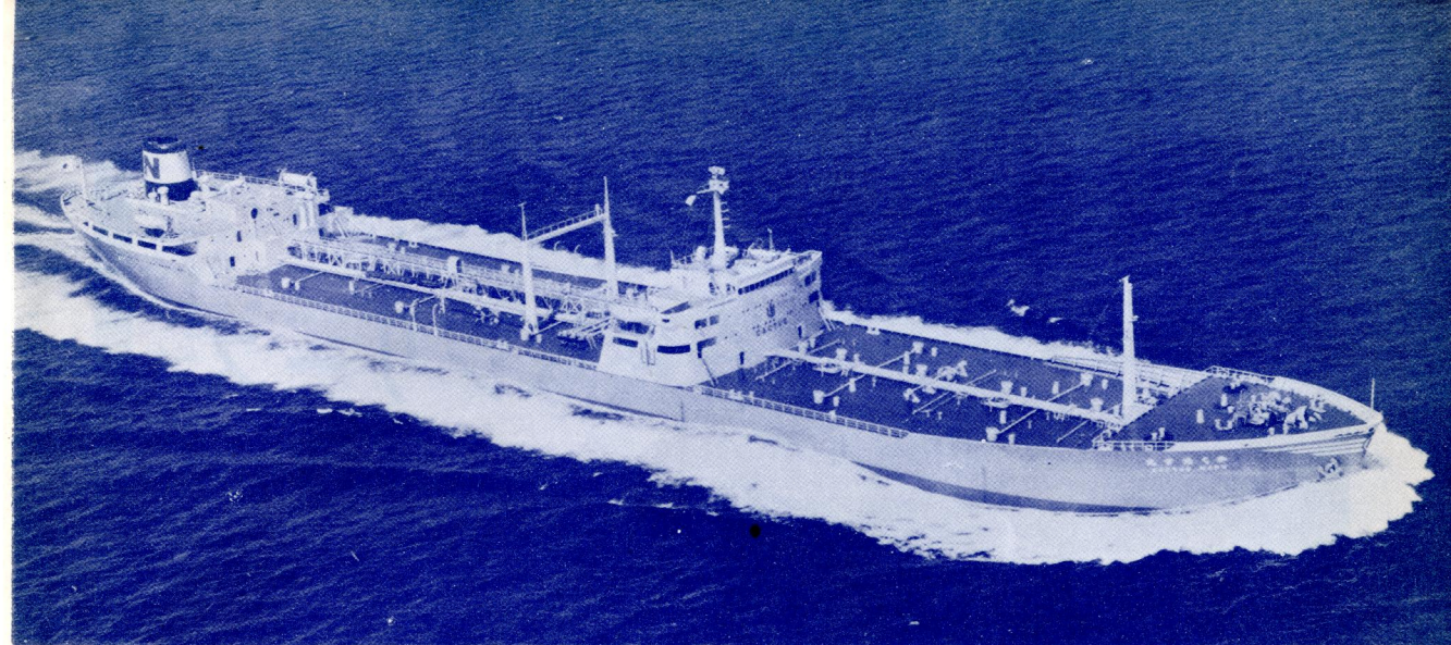
日正汽船の油槽船“かくたす丸”。三菱日本重工横浜造船所で6月29日完成。50,638重量トン、航海速力15.7ノット。
