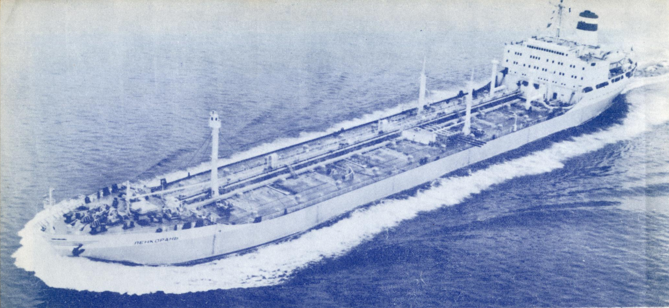
ソ連向け輸出タンカー“レンコラン” Lenkoran。石川島播磨重工相生第1工場で5月25日竣工。34,661重量トン、17ノット。
