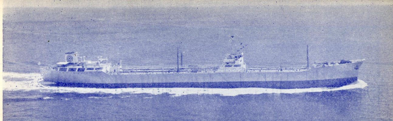
8月12日石川島播磨重工業相生第一工場で完成した三光汽船のタンカー「東光丸」。47,250 重量トン、航海速度16.2ノット
