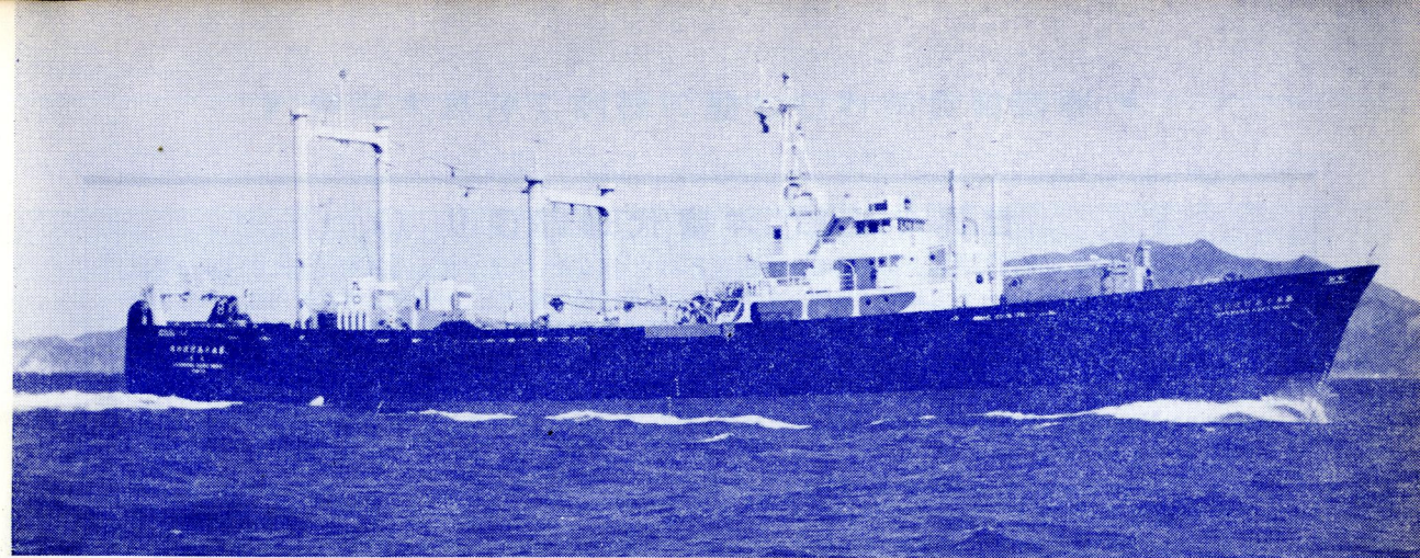
大型船尾式トロール船第五十あけほの丸(1,700重量トン)。日魯漁業の注文で三菱造船下関造船所が建造し、2月22日竣工した。
