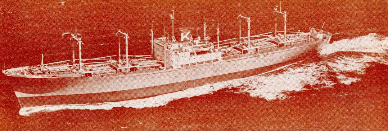
川崎重工で4月7日完成した川崎汽船ころらど丸。13,429重量トン、全長162.07メートル、最大速力21.23ノット
