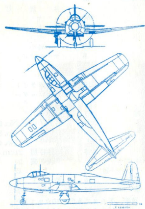
三面図見本・空技廠十八試陸偵「景雲」
