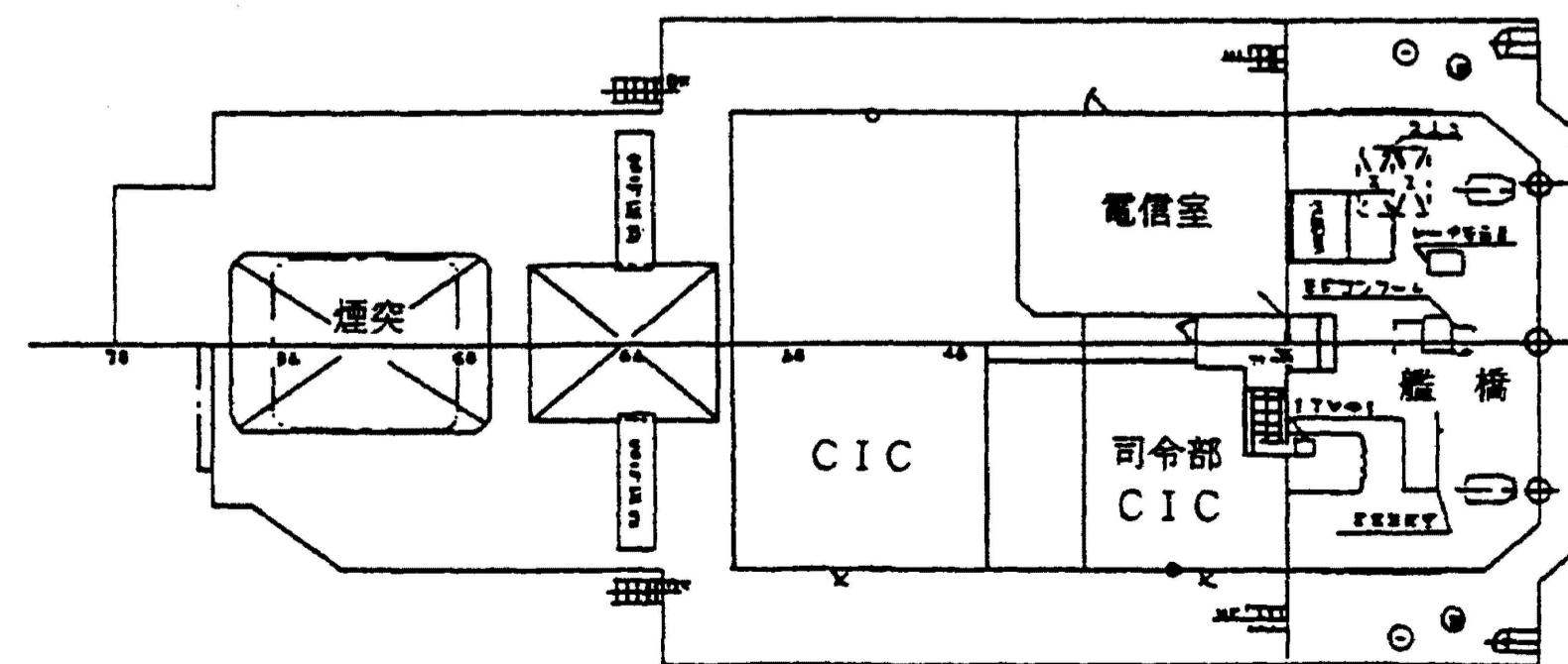
艦橋甲板
